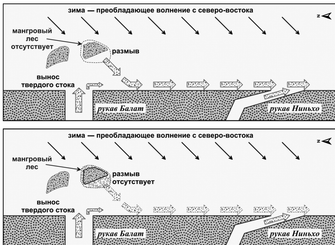
Рис. 4. Схема ослабления потока наносов мангровыми зарослями
