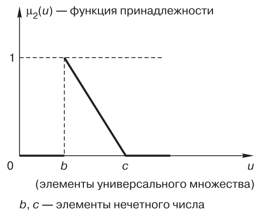
Рис. 3. График функции \mu_2(x)
