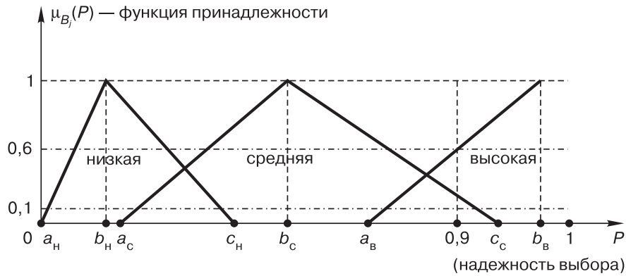
Рис. 5. Лингвистическая переменная «надежность выбора»
