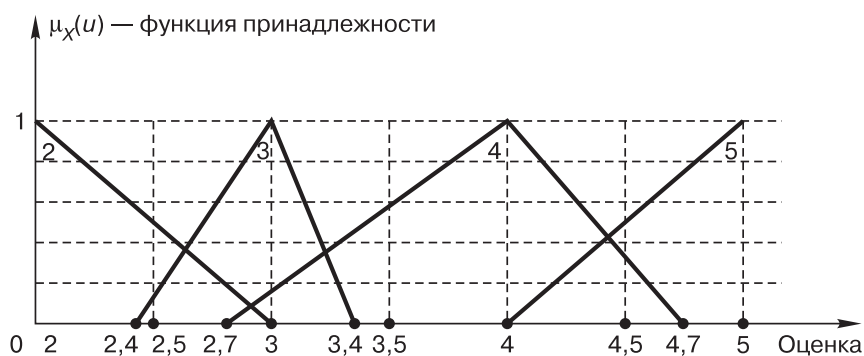
Рис. 6. Выходная лингвистическая переменная
