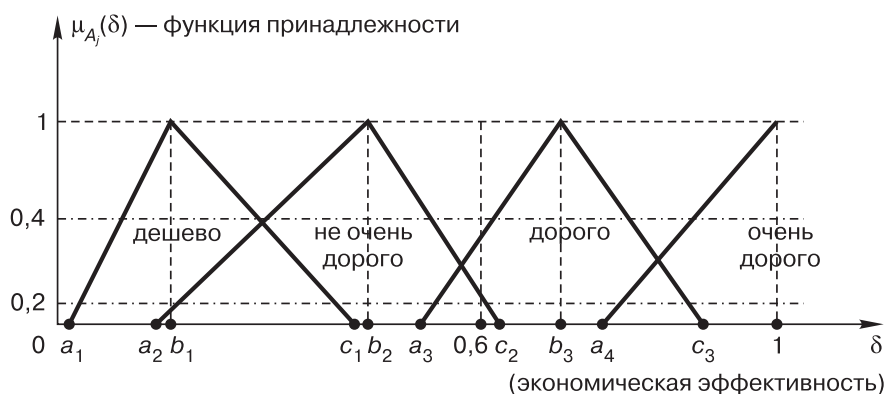
Рис. 4. Лингвистическая переменная «экономическая эффективность»
