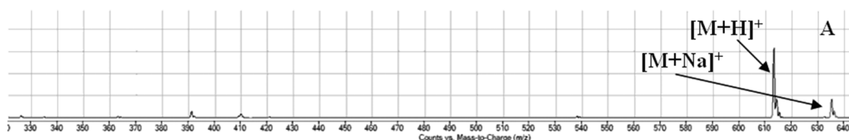
Рис. 3. Масс-спектр ИЭР «седатина»
