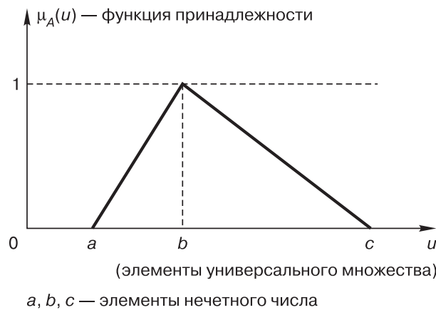
Рис. 1. Треугольное число
