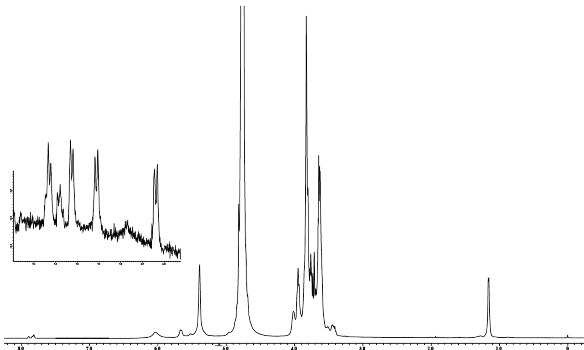
Рис. 2. Спектр ЯМР ^1\text{H} пленкообразующего раствора ЛС «седатина»
