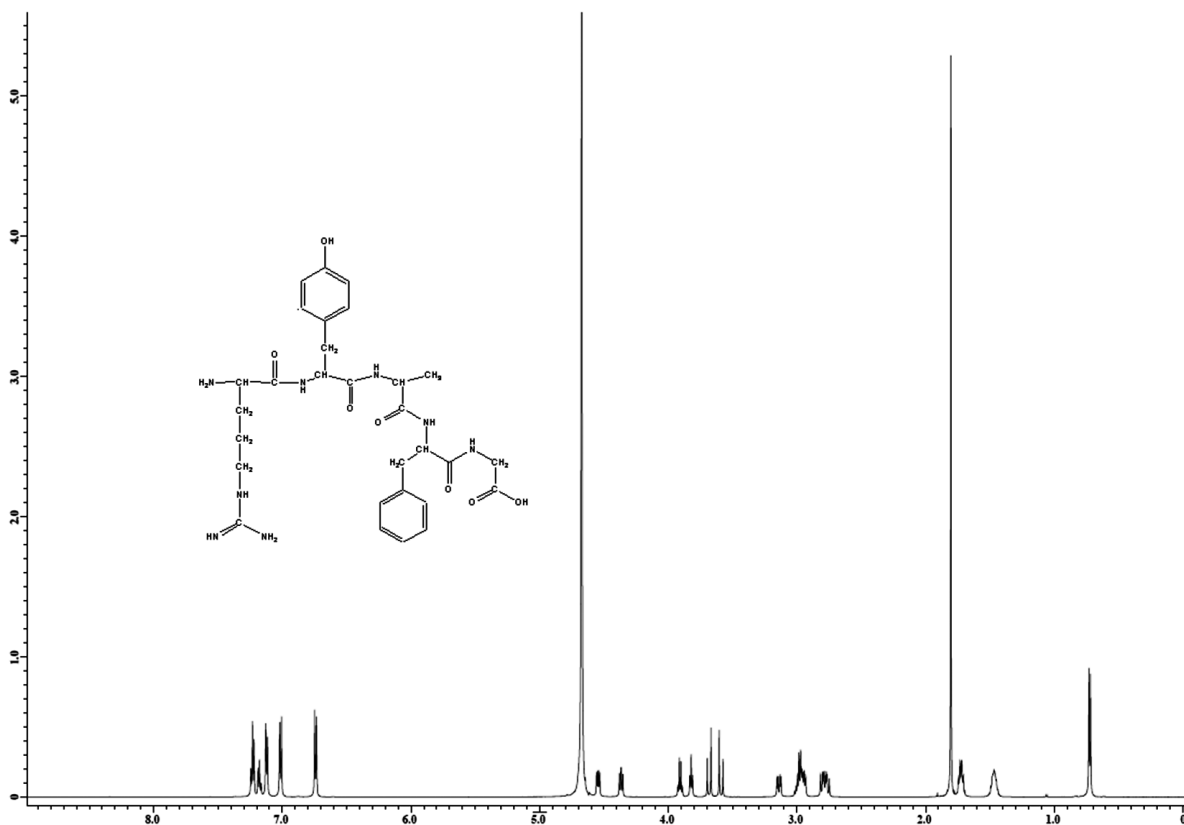
Рис. 1. Спектр ЯМР ^1H и формула «седатина»
