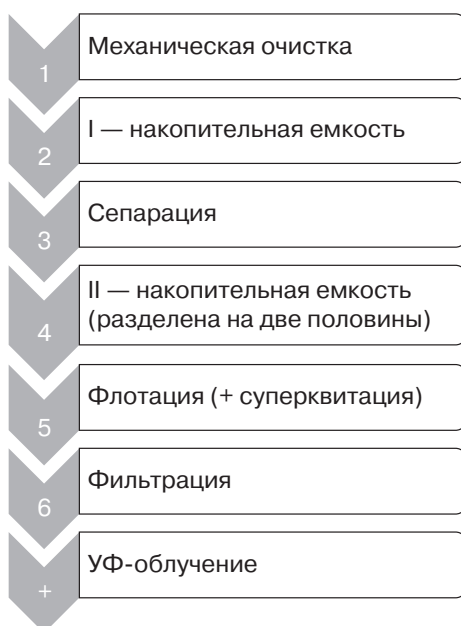
Рис. 1. Технологическая схема очистки сточных вод
